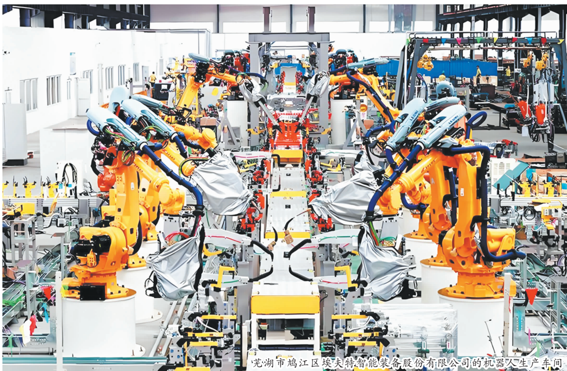
芜湖市鸠江区埃夫特智能装备股份有限公司的机器人生产车间。
